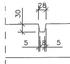
Detalje C
