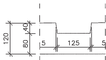
Detalje A
