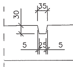
Detalje B
